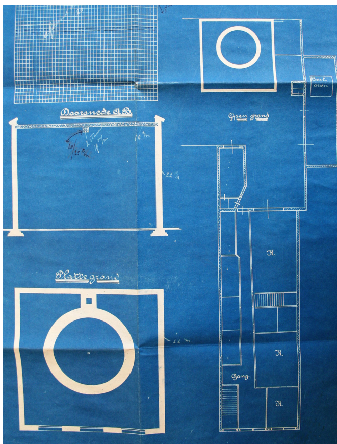
Afb. 62. Tekening bij aanvraag uitbreiding pijpenfabriek door C. de Rijk & Zoon. SAMH, ac 56, inv.nr. 1029.
