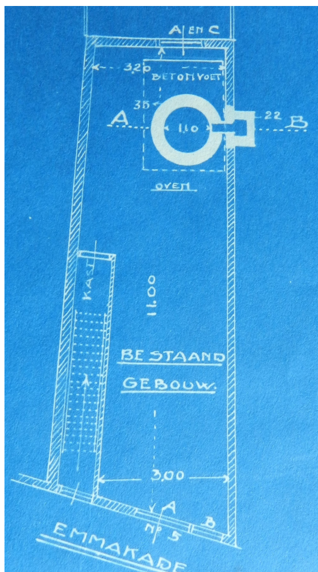
Afb. 48a-b. Plattegrond met oven. Tekening bij aanvraag Hinderwetvergunning Emmakade 5, Haarlem.
