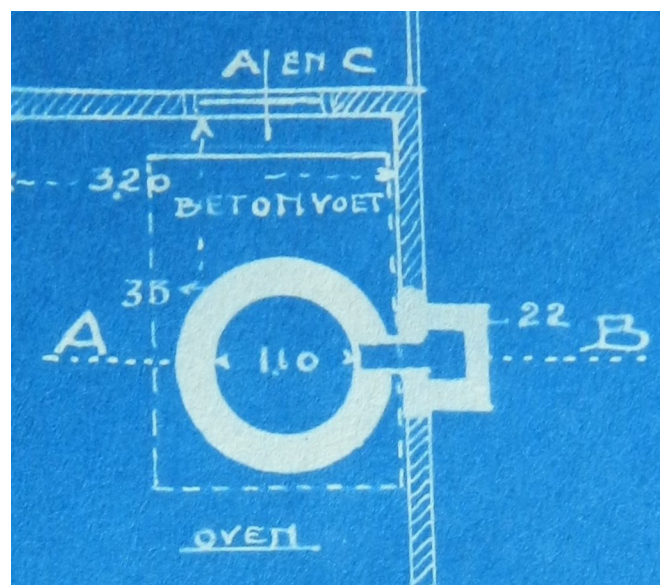
Afb. 48a-b. Plattegrond met oven. Tekening bij aanvraag Hinderwetvergunning Emmakade 5, Haarlem.
