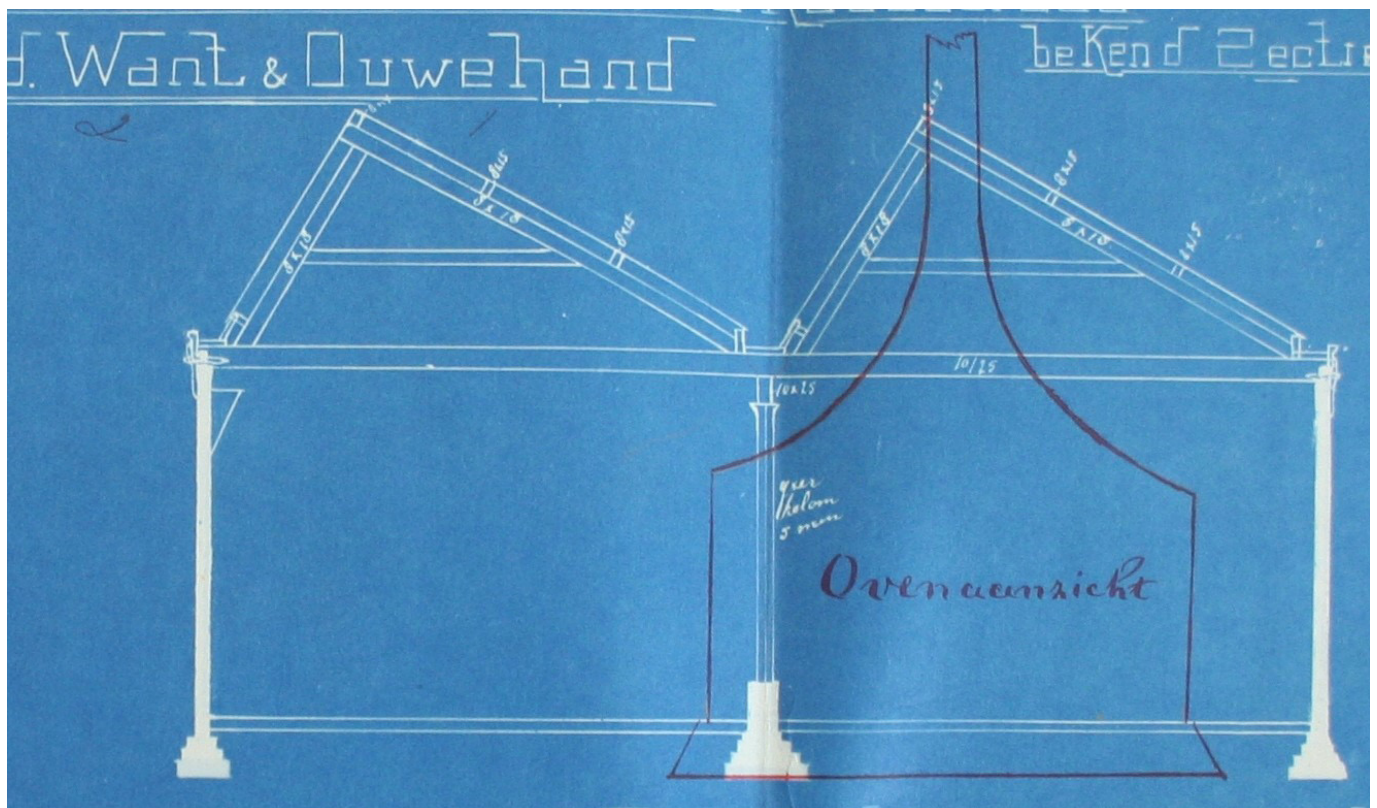
Afb. 58. Lage Gouwe 140 blauwdruk met oven en ovenhuis voor Neerlandia, mei 1915.
